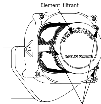
Vis de retenue
