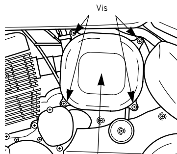
Couvercle du filtre a air
